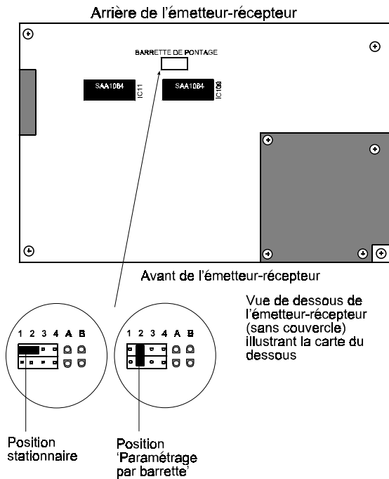
Figure 9.1 Repositionnement de la barrette en mode 'Paramétrage par barrette de pontage'
