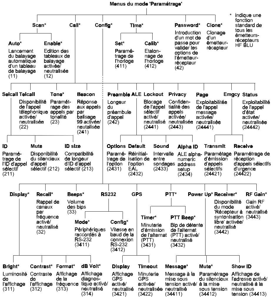
Figure 4.1 Arbre du mode Paramétrage
