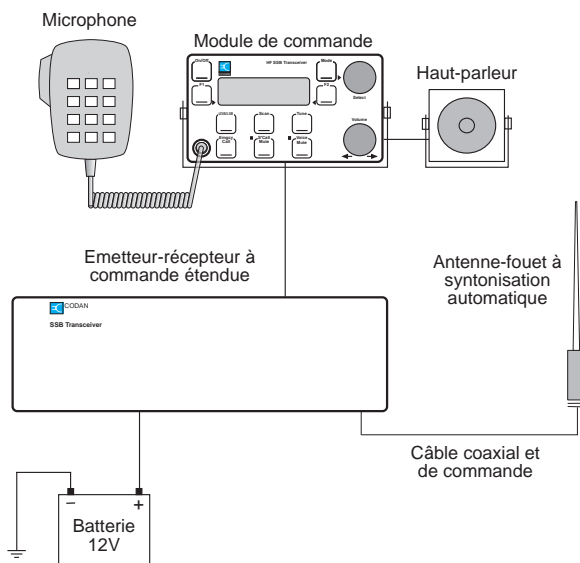
Figure 2.2 Poste mobile typique
