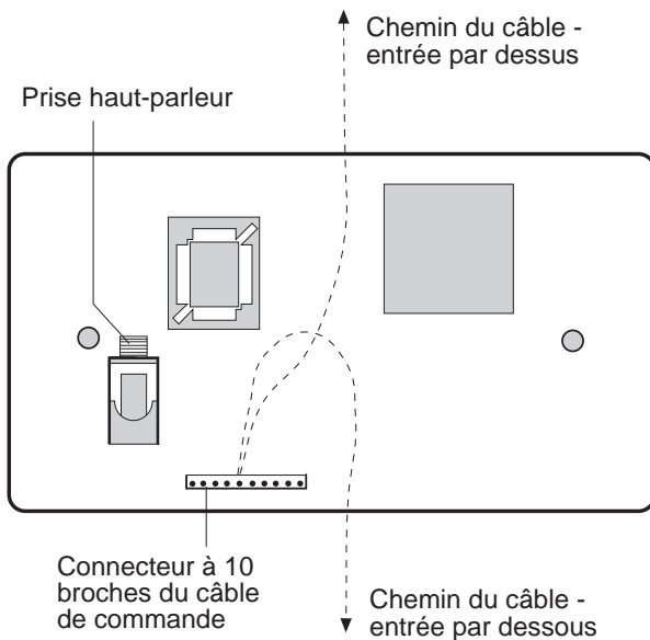
Figure 2.3 Vue arrière du module de commande sans couvercle
