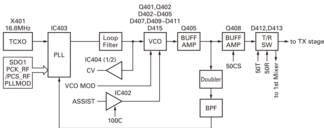
Fig. 6 PLL block diagram / 图 6 PLL 结构图
