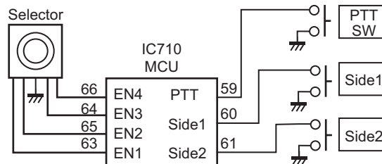
Fig.8 Key input
