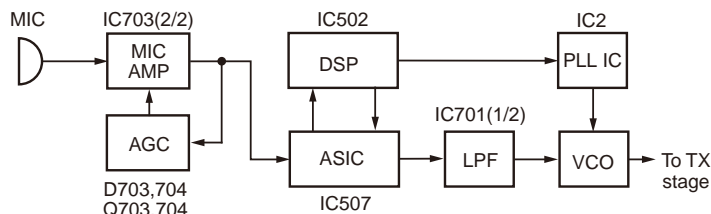
Fig. 4 Transmitter System / 图 4 发射机系统
