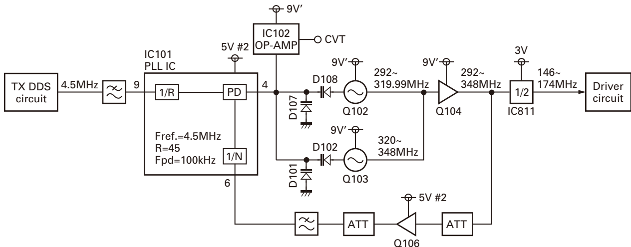
Fig. 5 Transmitter main PLL circuit / 图5 发射机主 PLL 电路
