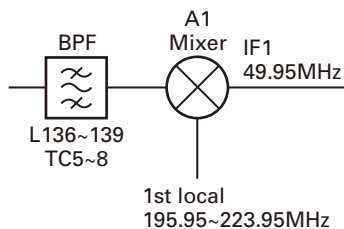
Fig. 17 1st-Mixer circuit / 图 17 第 1 混频器电路
