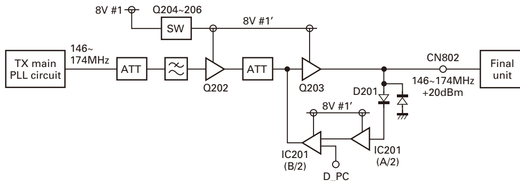
Fig. 6 Driver circuit / 图 6 驱动电路
