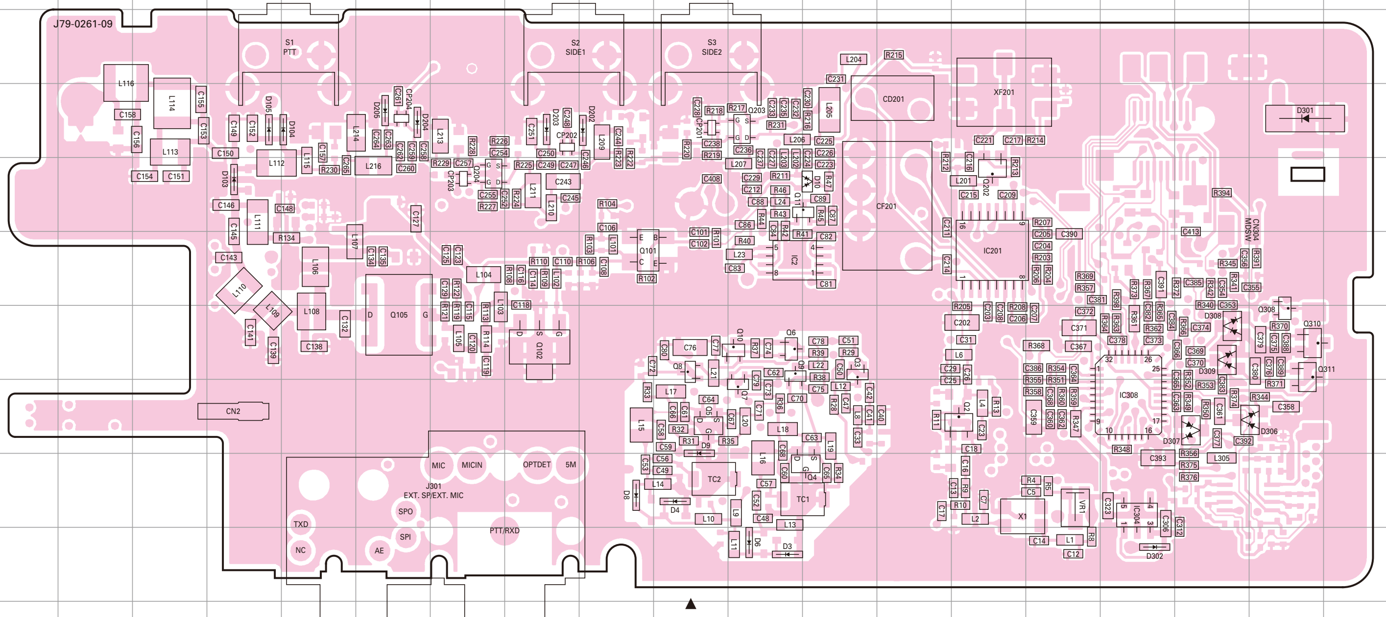
TX-RX UNIT (X57-7572-71) Foil side view (J79-0261-09)
