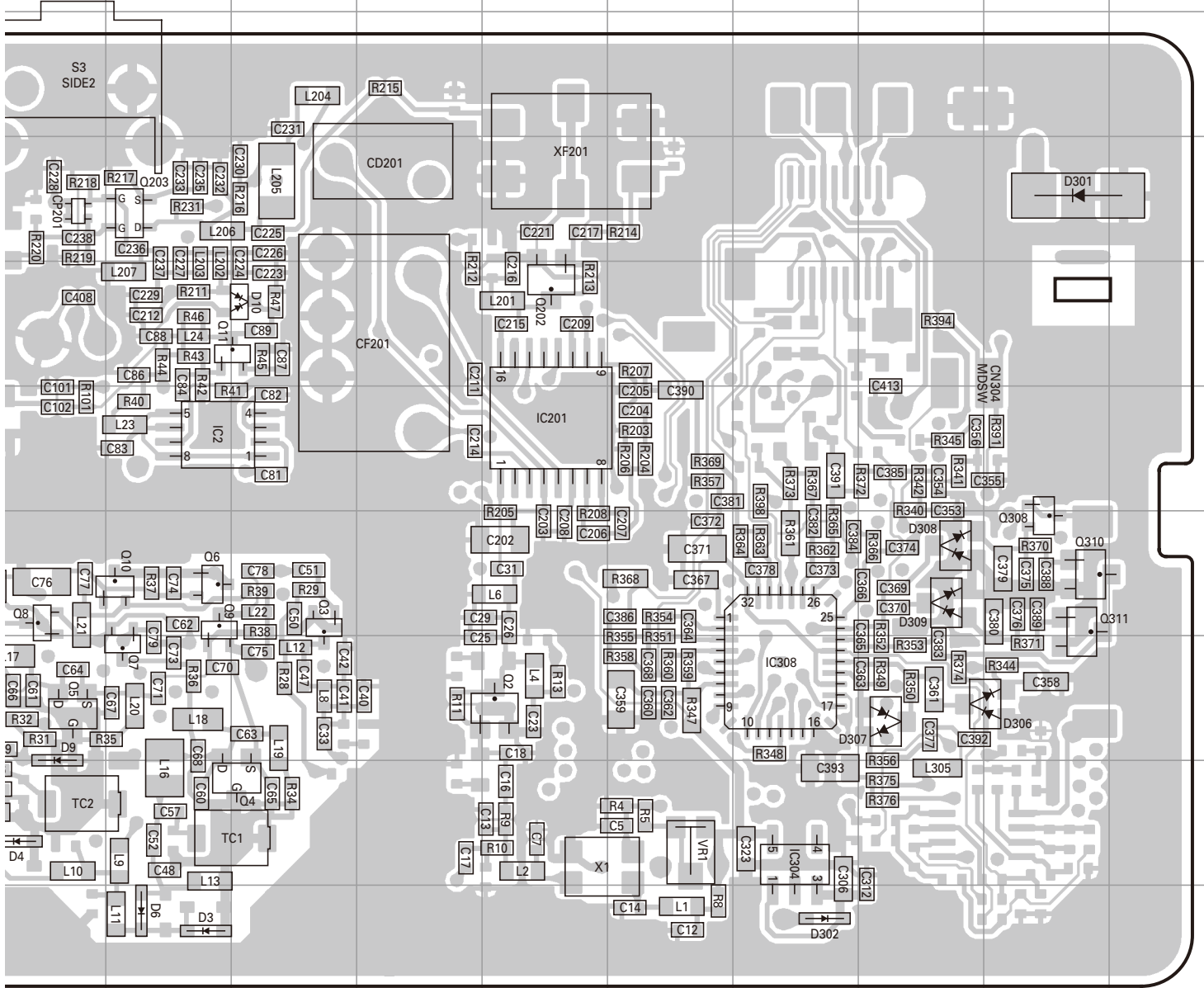
TX-RX UNIT (X57-7572-71) Foil side view (J79-0261-09)
