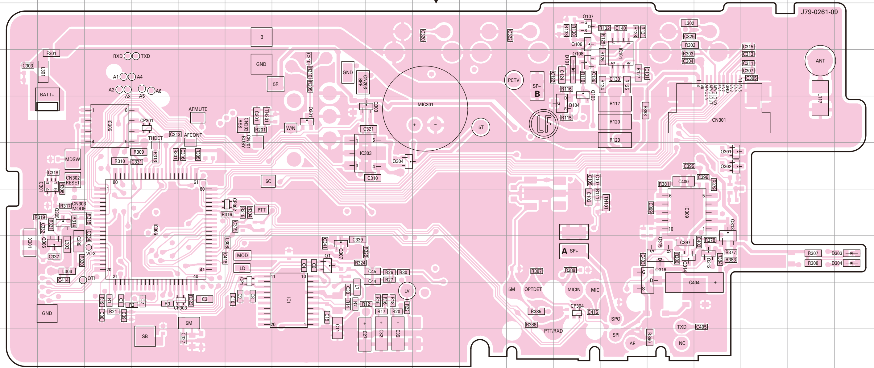
TX-RX UNIT (X57-7572-71) Component side view (J79-0261-09)
