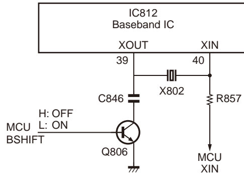
Fig. 7 Frequency shift circuit / 图 7 频率偏移电路
