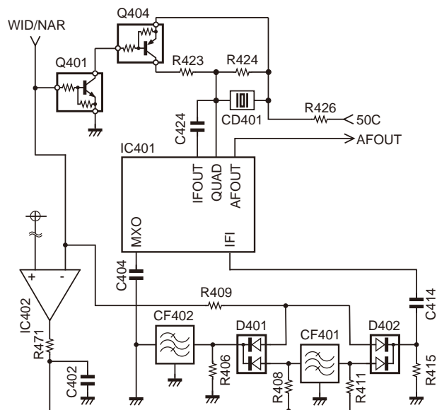
Fig. 3 Wide/Narrow switching circuit / 图 3 宽 / 窄切换电路
