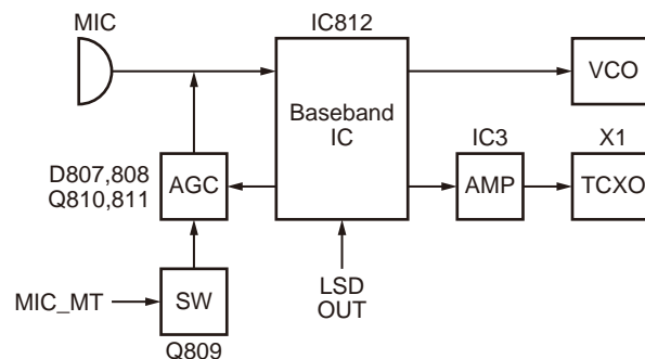
Fig. 4 Microphone amplifier circuit / 图 4 麦克风放大器电路
