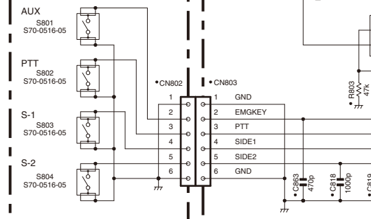
TX-RX UNIT (X57-7782-71(B)3)
