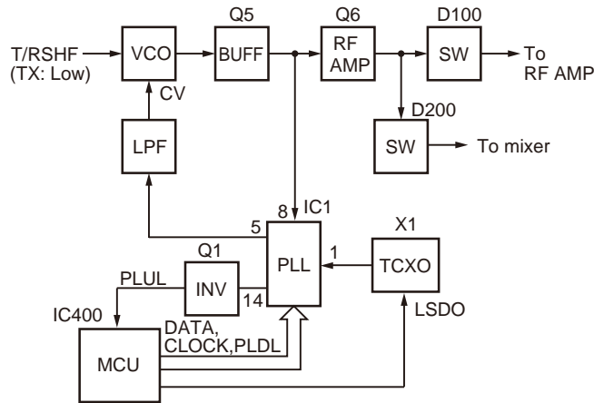
Fig. 5 PLL block diagram / 图 5 PLL 方块图
