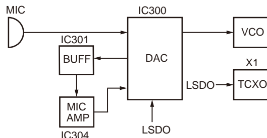
Fig. 3 Microphone amplifier circuit / 图3 麦克风放大器电路
