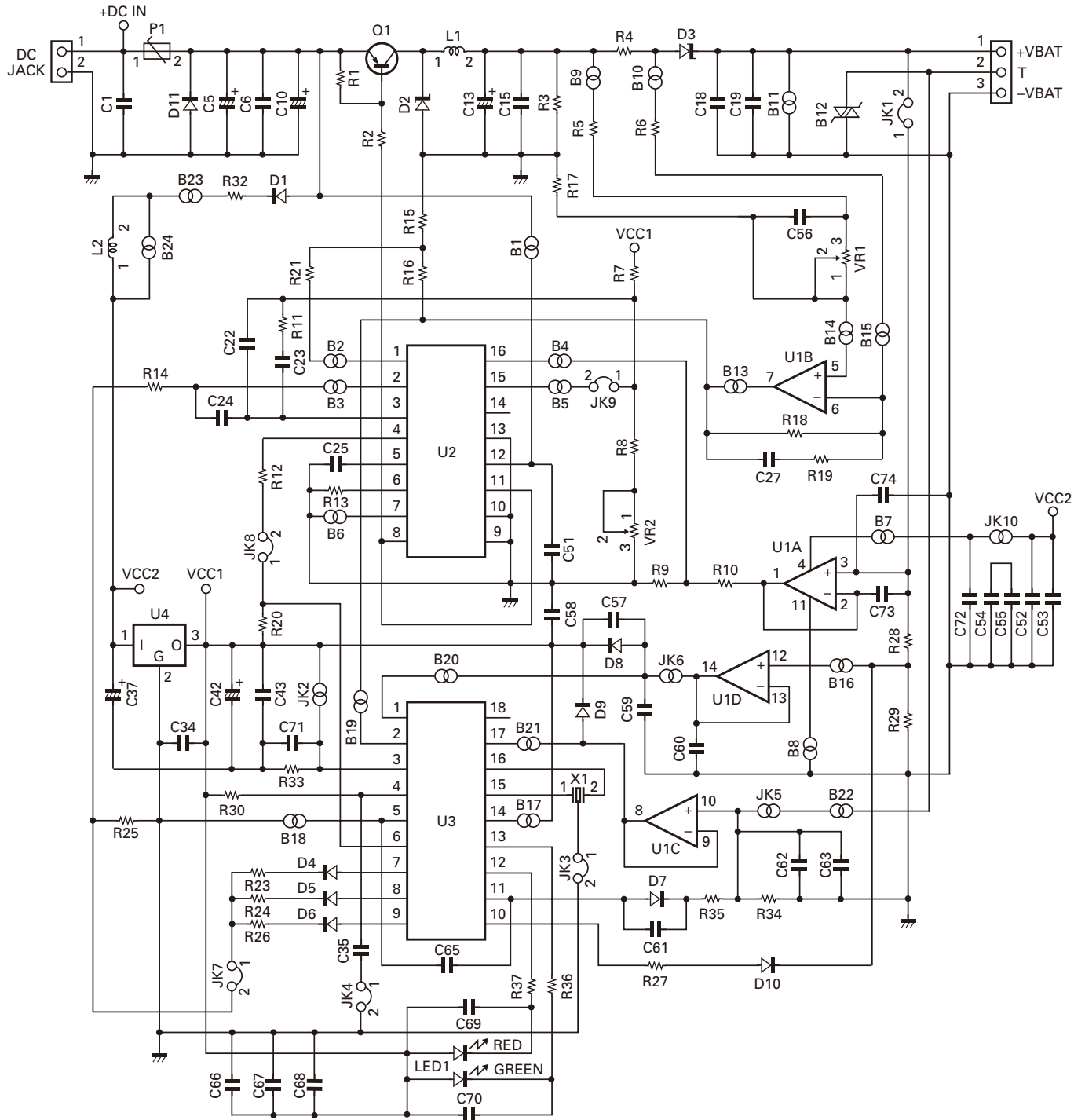
■ Schematic Diagram / 原理图
