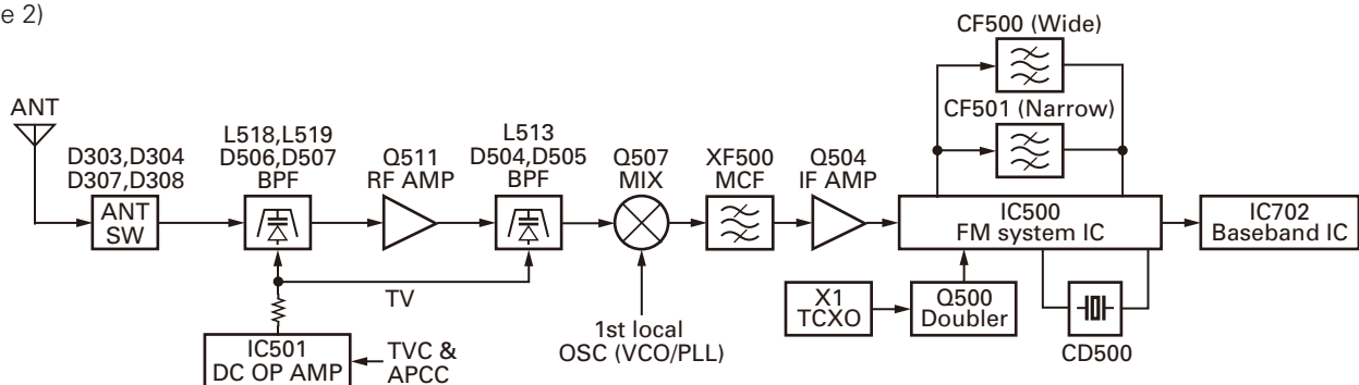
Fig. 2 Receiver System / 图 2 接收机系统
