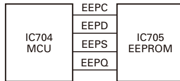
Fig. 11 Memory circuit / 图 11 存储电路
