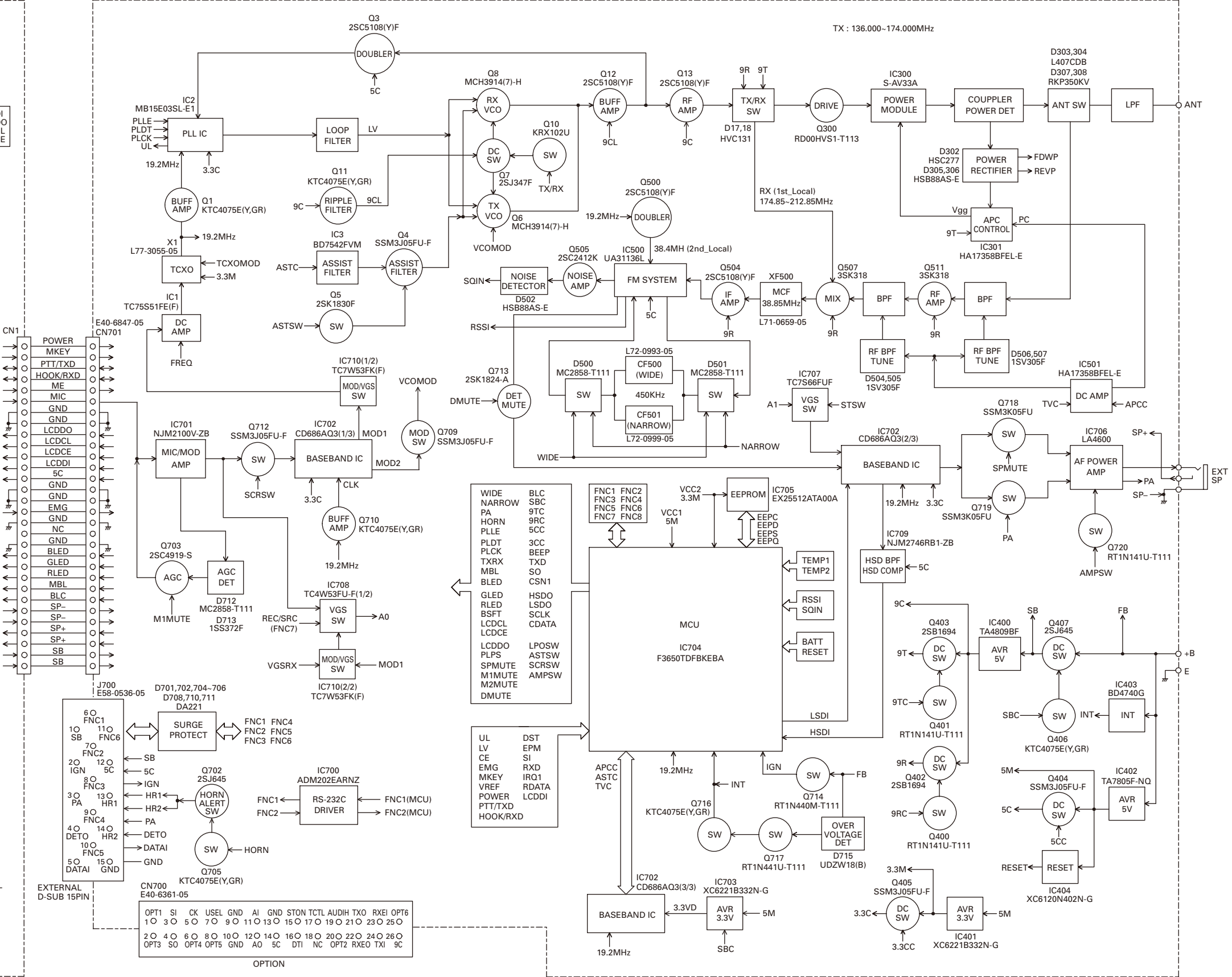
TX-RX UNIT (X57-802)
