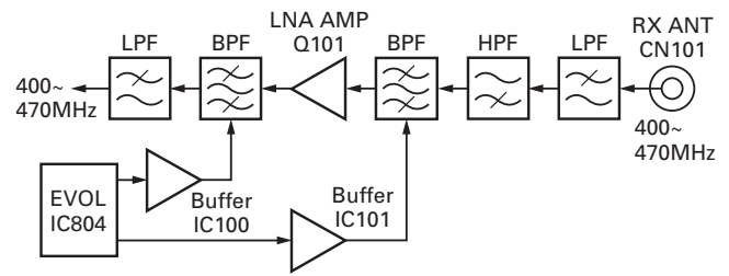
Fig. 6 Front-end circuit
