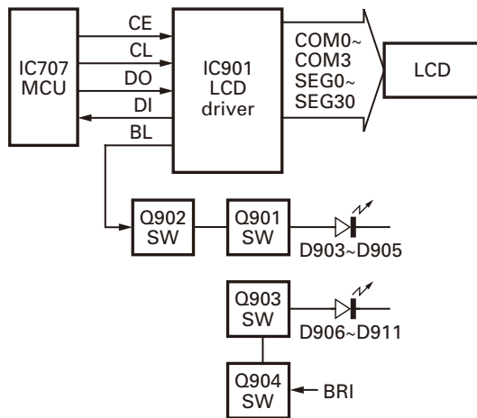
Fig. 12 Display circuit
