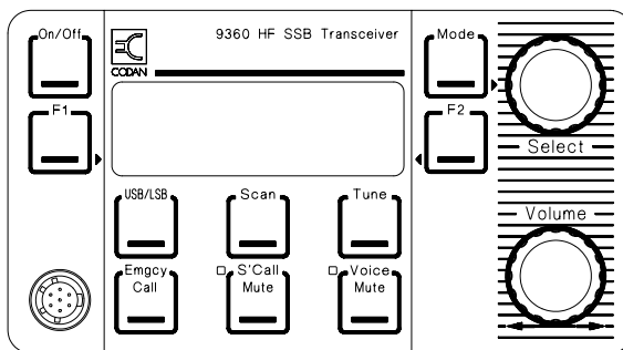
Figure 2-4: Module de commande étendue (9366) de l'émetteur-récepteur HF BLU 9360
