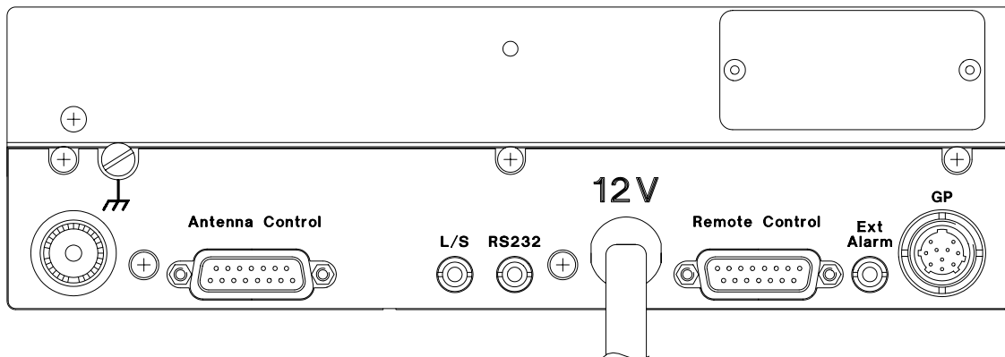
Figure 2-8: Face arrière des émetteurs-récepteurs HF BLU 9323, 9360, 9390 et 9780
