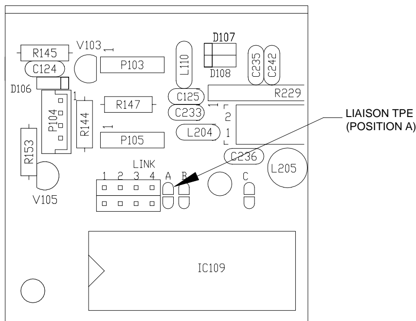
Figure 6-1: Extrait de la carte Microprocesseur et Audio
