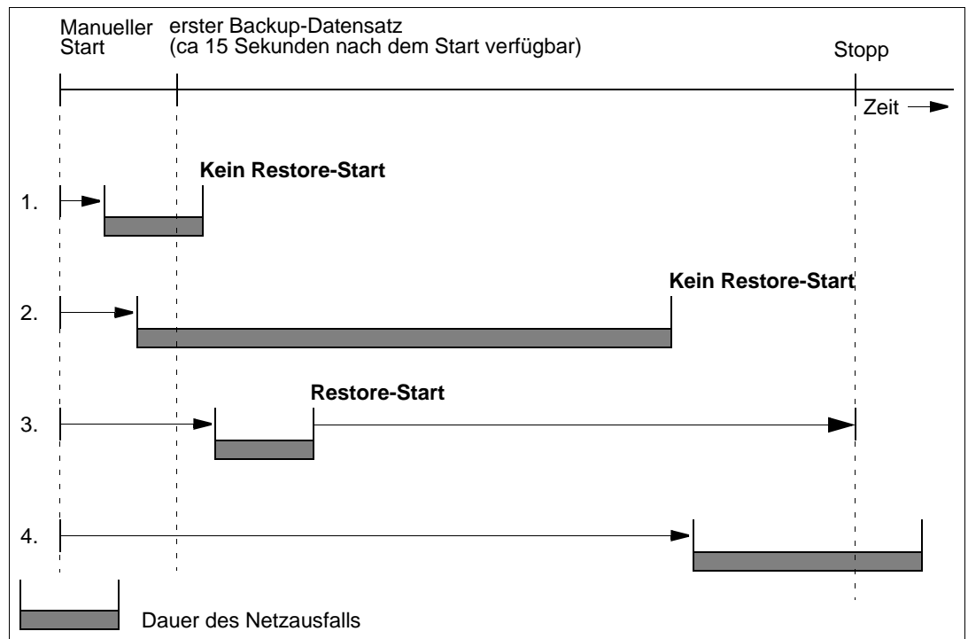
Bild B-40 Beispiele für das Verhalten des ANT-20SE bei Netzausfall (manuell gestartete Messungen)
