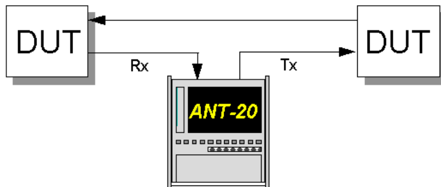
Bild A-8 Monitoring mit eingeschleiftem ANT-20SE
