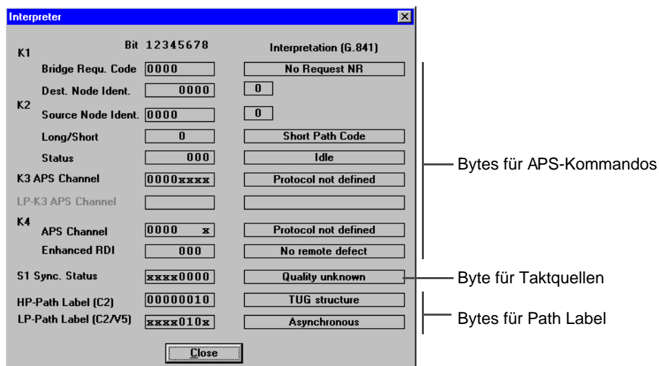
Bild VI-22 Fenster "Interpreter" zur Klartextanzeige von SOH/POH-Bytes
