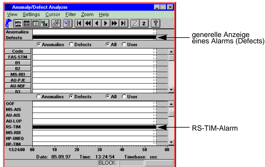
Bild A-49 Fenster "Anomaly/Defect Analyzer"
