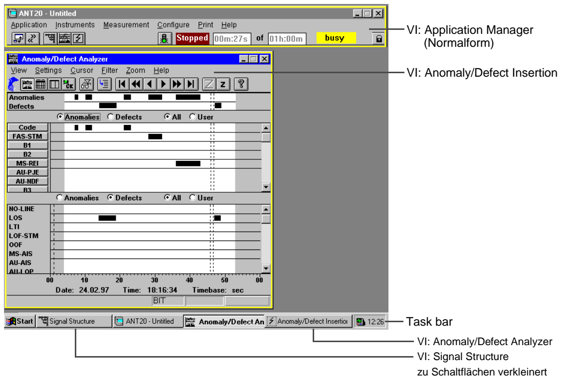
Bild B-31 Bildschirmdarstellung der virtuellen Instrumente
