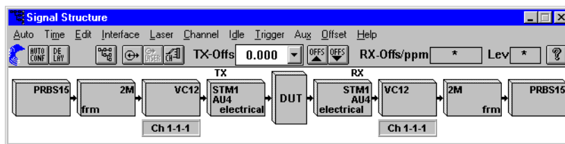
Bild B-20 Fenster "Signal Structure" nach der Eingabe der Signalstruktur
