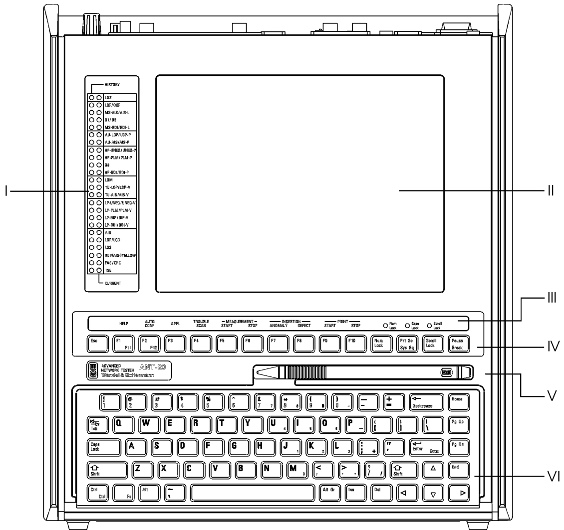
Bild B-1 Frontseite des ANT-20SE
