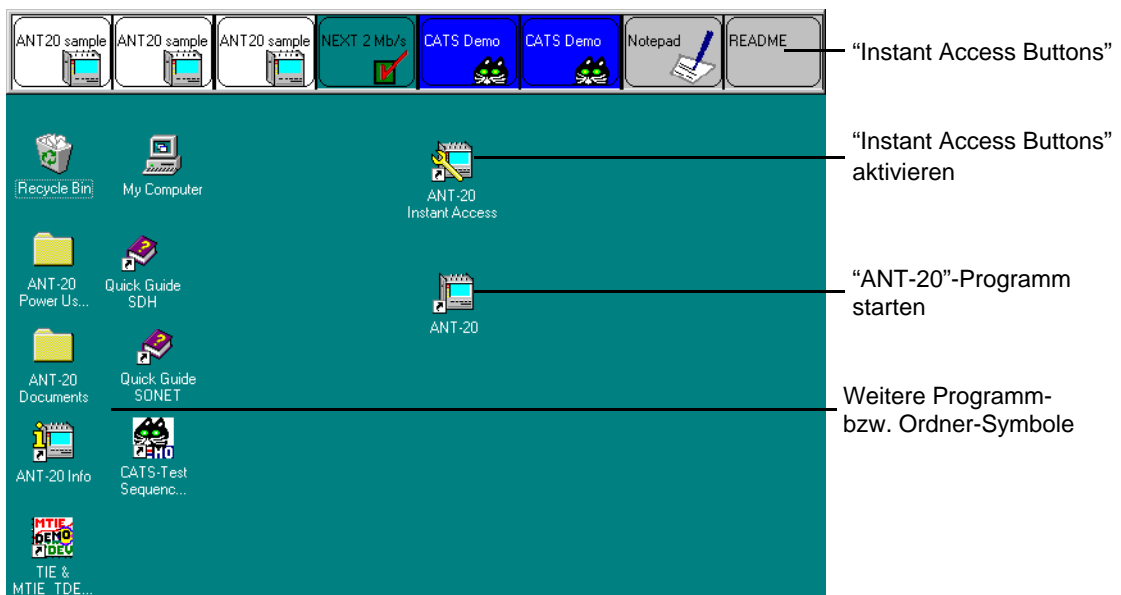
Bild B-5 Desktop des ANT-20SE nach Aktivierung der "Instant Access Buttons"
