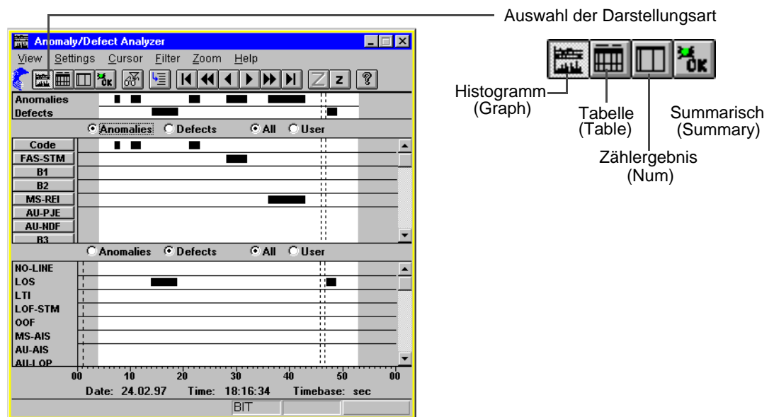
Bild B-29 Beispiel einer Ergebnisanzeige im Fenster "Anomaly/Defect Analyzer" (View "Graph")
