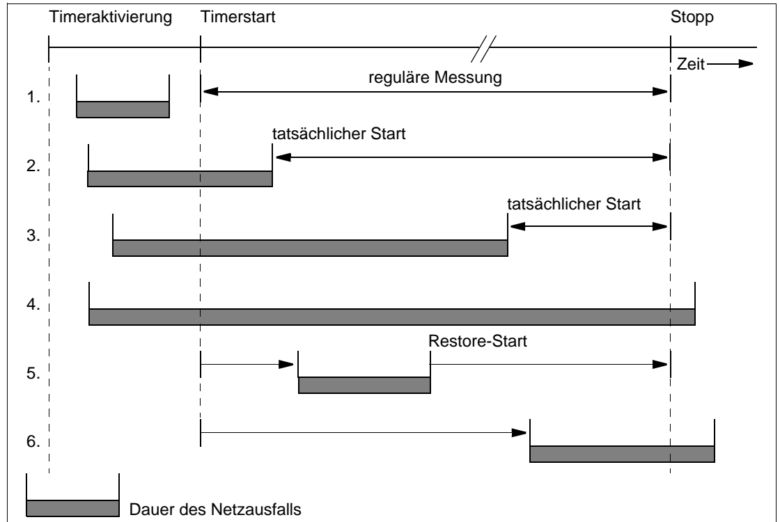
Bild B-41 Beispiele für das Verhalten des ANT-20SE bei Netzausfall ("Timer"-gestartete Messungen)
