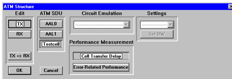
Bild A-95 Dialog "ATM Structure" des VIs "ATM Signal Structure"
