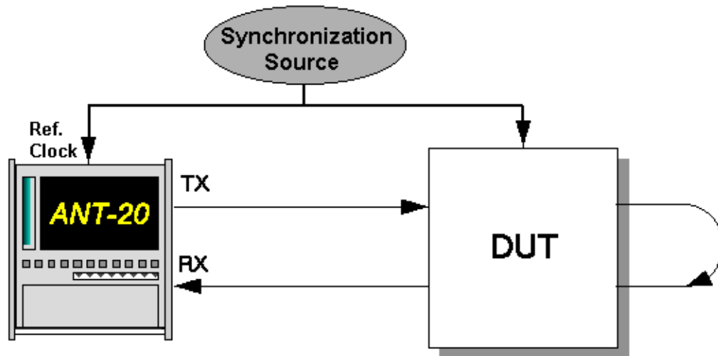
Bild A-73 Meßaufbau für Wanderverträglichkeitsmessungen
