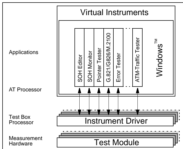
Bild E-3 Software-Architektur des ANT-20SE
