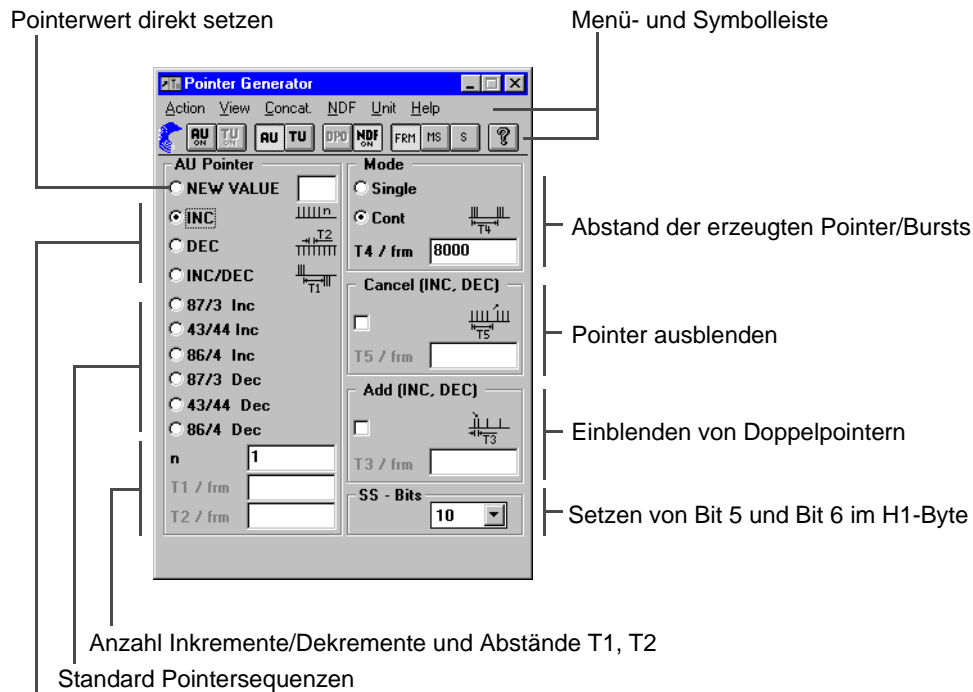
Bild VI-25 Elemente des Hauptfensters "Pointer Generator"
