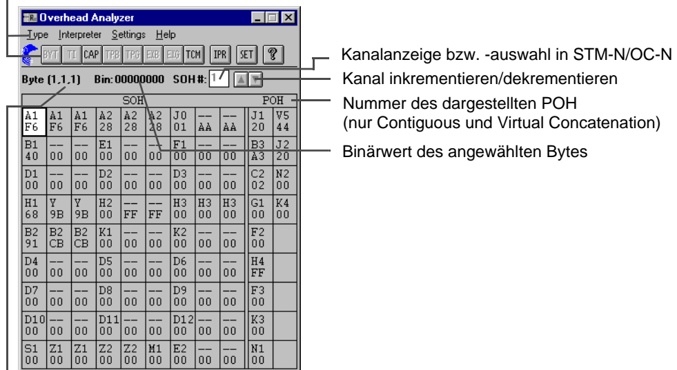
Bild VI-21 Elemente des Hauptfensters "Overhead Analyzer"
