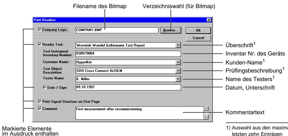
Bild B-35 Dialog "Print Headers"
