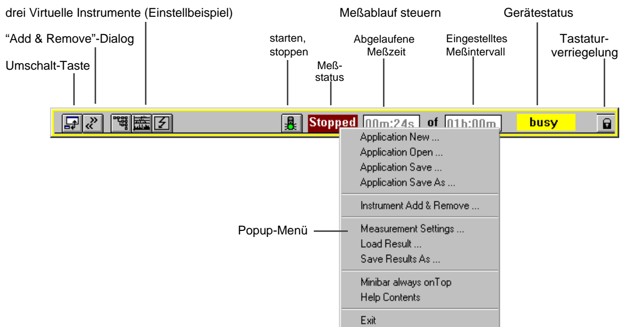
Bild B-7 Die Bereiche der Symbolleiste bzw. “Minibar” des Fensters “ANT20 - <Application Title>”
