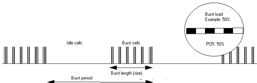
Bild A-125 Defintion der Burst period, Burst length etc.
