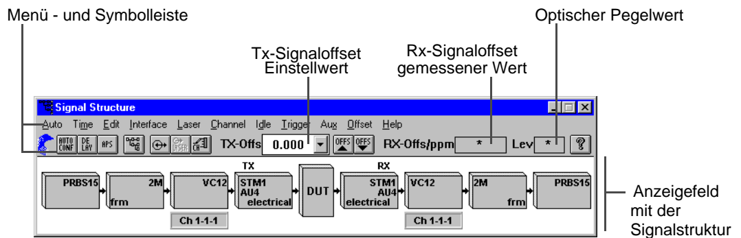
Bild VI-1 Elemente des Hauptfensters "Signal Structure"
