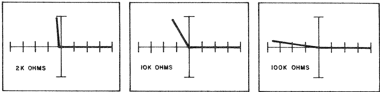
2K-OHM RESISTOR
